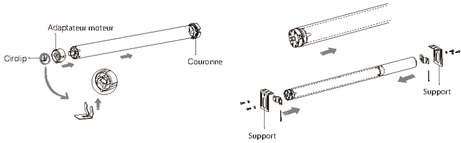
Etape 3 : Installer la couronne et l'adaptateur moteur. Assurez vous que l'adaptateur s'adapte fermement et que la couronne tourne librement.
