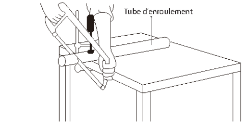
Etape 1 : Recouper le tube d'enroulement
